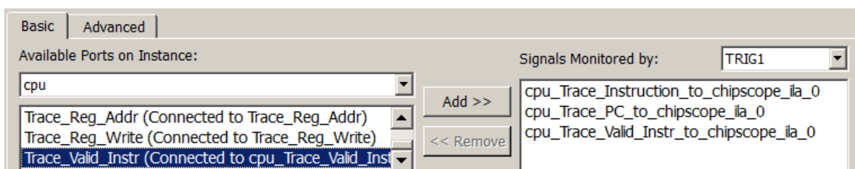
Abbildung 5: Verbindung der Trace-Signale mit »TRIG1«
